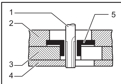
► 1. Fresa 2. Base 3. Plantilla 4. Pieza de trabajo 5. Guía de plantilla
