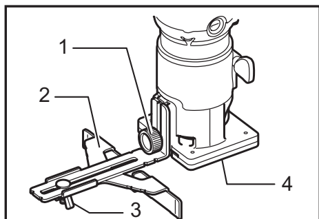
► 1. Tornillo de sujeción (A) 2. Guía recta 3. Tuerca de mariposa 4. Base
