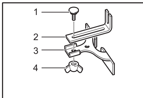
► 1. Bolt 2. Guide plate 3. Straight guide 4. Wing nut
