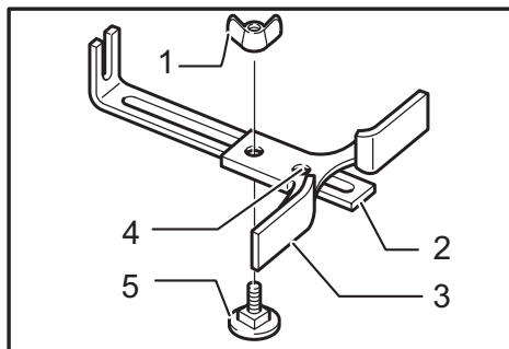
► 1. Wing nut 2. Guide plate 3. Straight guide 4. Center hole 5. Bolt
