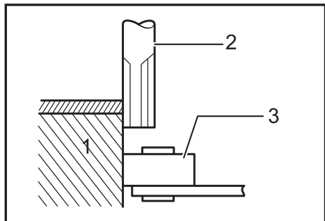
► 1. Pièce 2. Embout 3. Rouleau-guide
