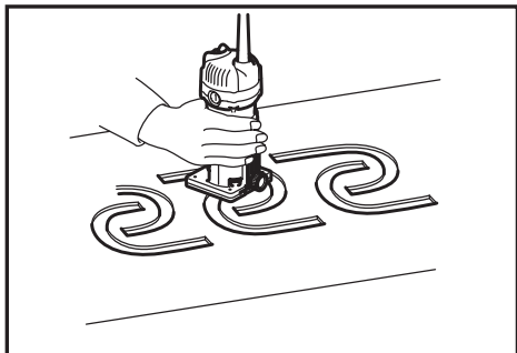
► 1. Fresa 2. Base 3. Plantilla 4. Pieza de trabajo 5. Guía de plantilla
