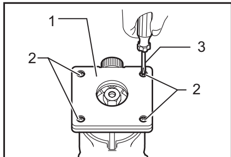
► 1. Protector de la base 2. Tornillos 3. Destornillador
