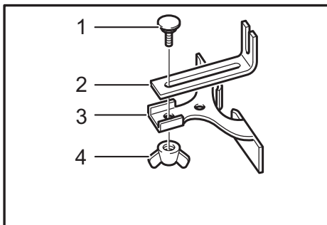
► 1. Perno 2. Placa guía 3. Guía recta 4. Tuerca de mariposa
