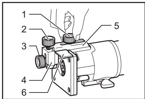
► 1. Vis de serrage (A) 2. Vis de réglage 3. Vis de serrage (B) 4. Guide d'affleurage 5. Porte-guide 6. Déflecteur de copeaux
